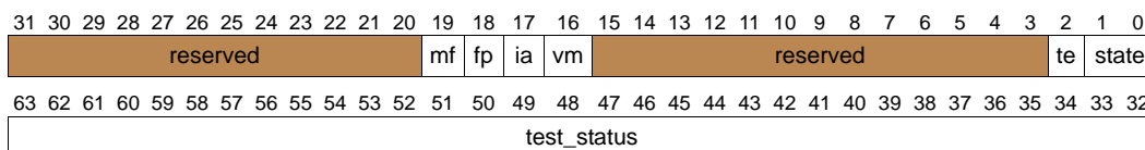
Figure 11-10. Self Test State Parameter
