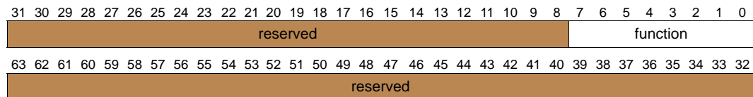
Figure 11-15. SALE_ENTRY State Parameter
