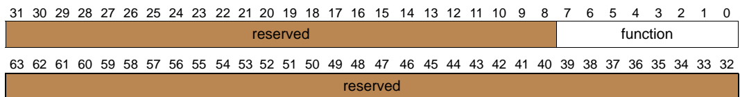
Figure 11-17. SALE_ENTRY State Parameter
