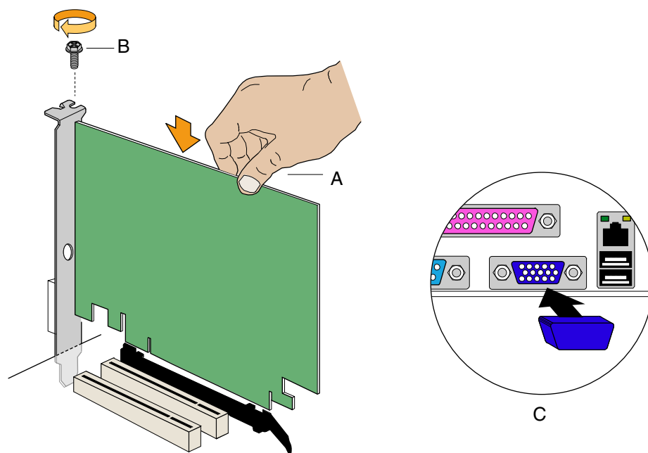
图 17. 插入 PCI Express x16 卡并盖好背面板 VGA 端口
