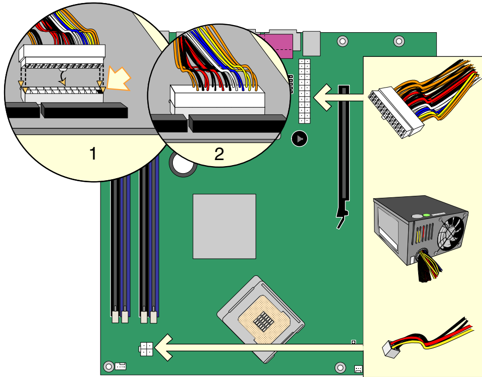
图 23. 连接电源系统电缆
