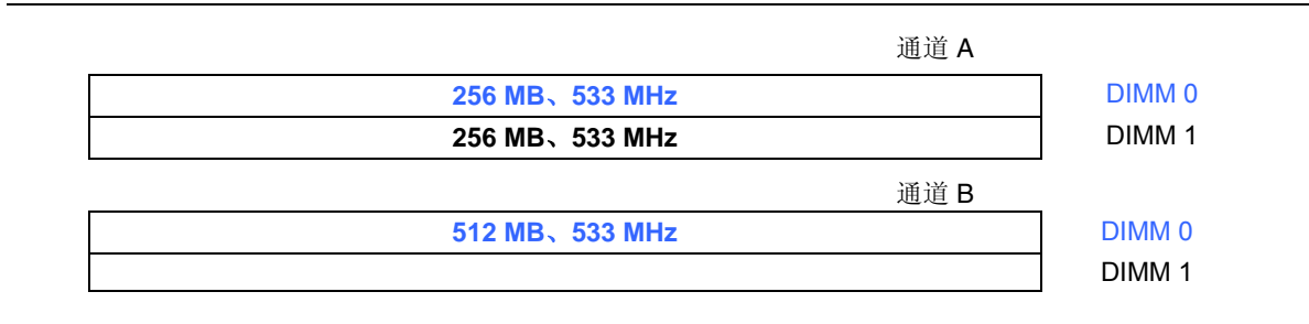
图 15. 双通道配置示例 3
