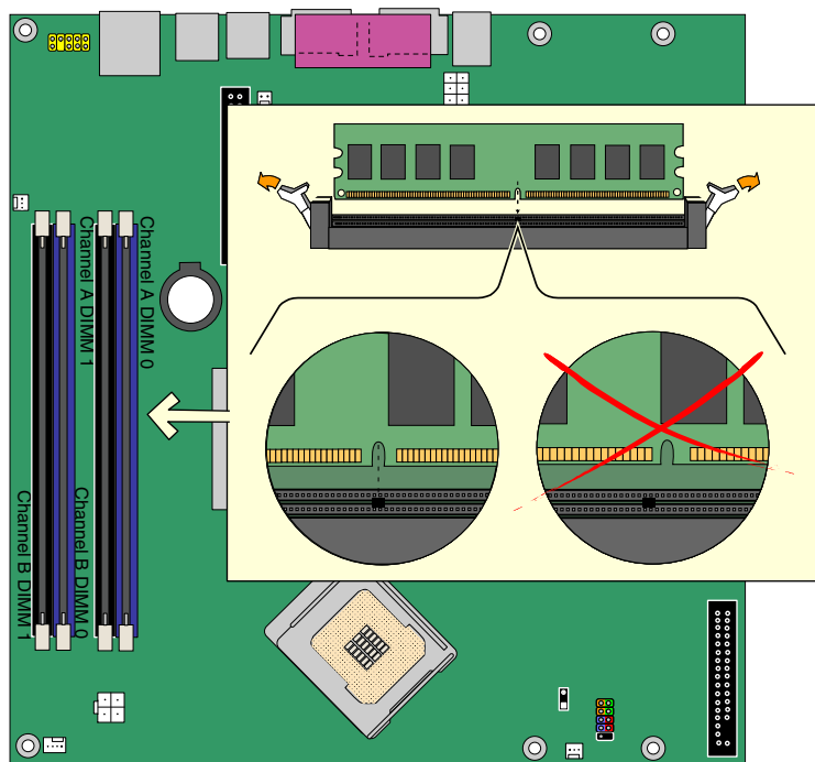
图 16. 安装 DIMM
