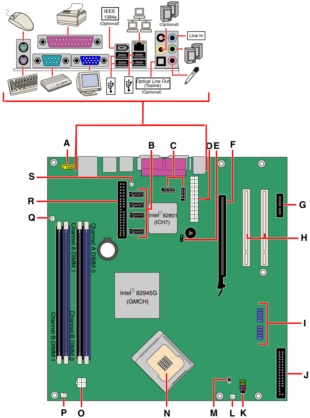
图 1. 桌面主板 D945GCZ 组件
