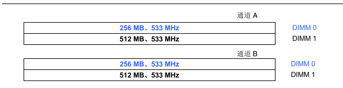
图 14. 双通道配置示例 2
