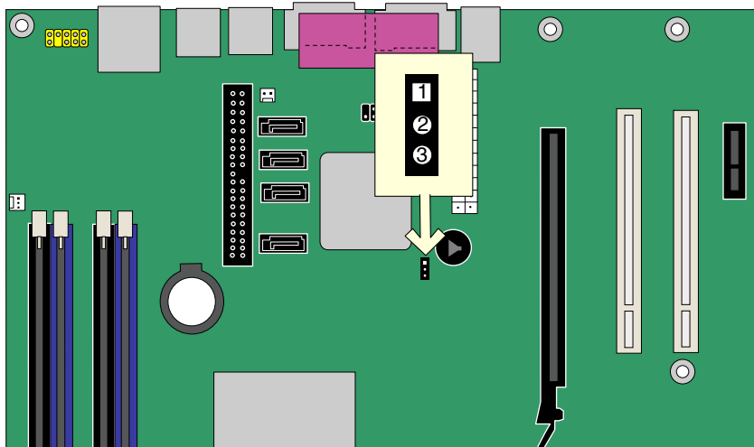
图 25. BIOS 配置跳线位置
