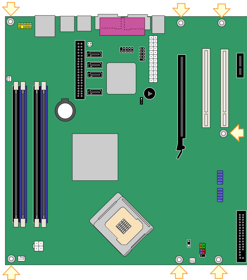
图 5. 桌面主板 D945GCZ 安装螺丝孔位置
