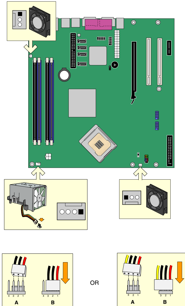
图 22. 风扇接头连接器位置
