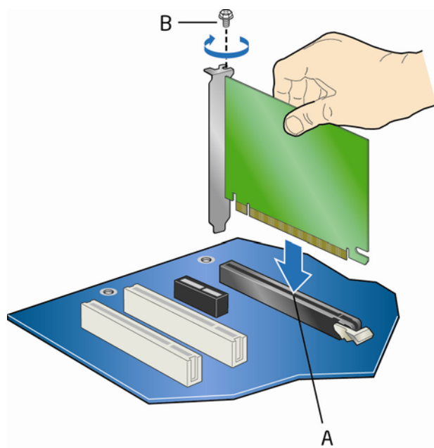
图 18. 安装 PCI Express x16 卡
