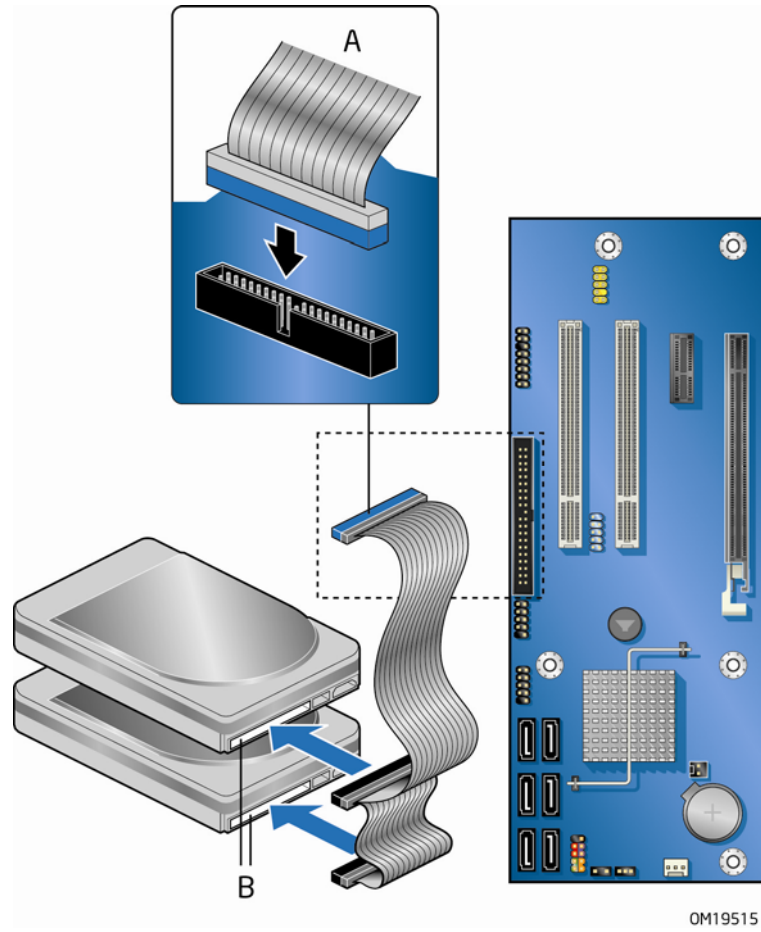
图 20. 连接 IDE 电缆
