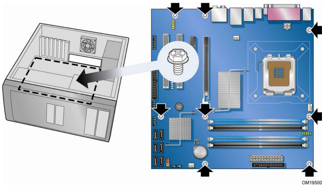
图 5. 台式机主板 DG965OT 安装螺丝孔位置
