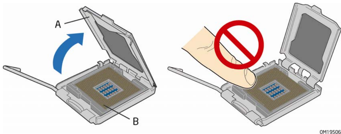
图 7. 抬起压板
