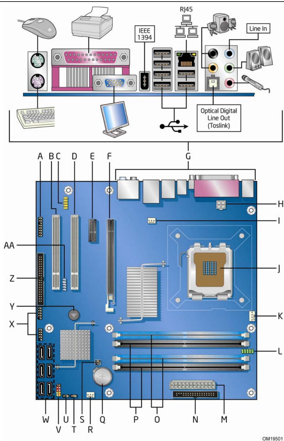
图 1. 台式机主板 DG965OT 组件
