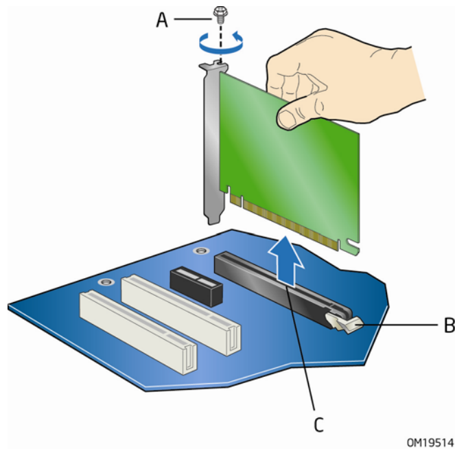
图 19. 拆卸 PCI Express x16 卡
