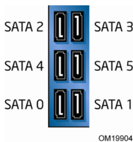
图 31. 启用 RAID 后台式机主板 DG965OT SATA 端口映射
