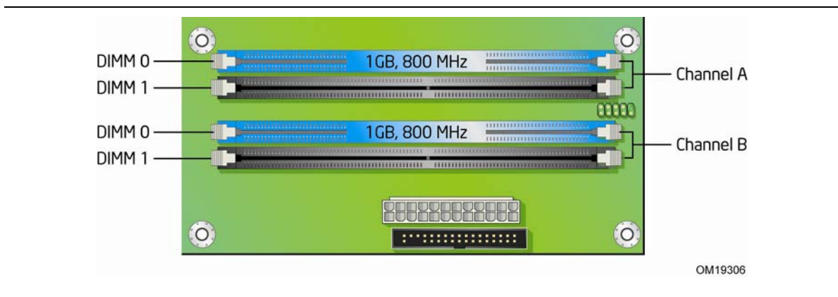
图 13. 双通道内存配置示例 1
