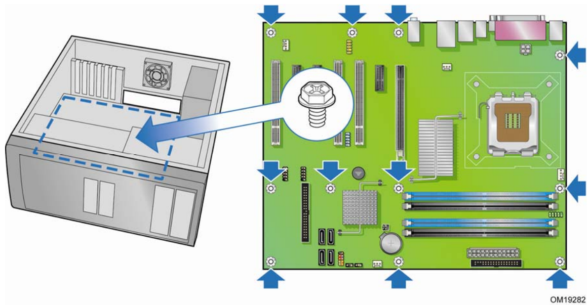
图 5. 台式机主板 DG965RY 安装螺丝孔位置
