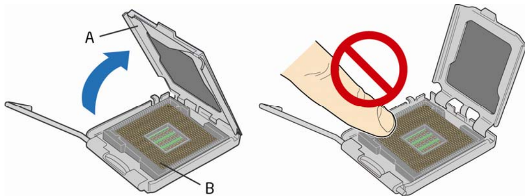
图 7. 抬起压板
