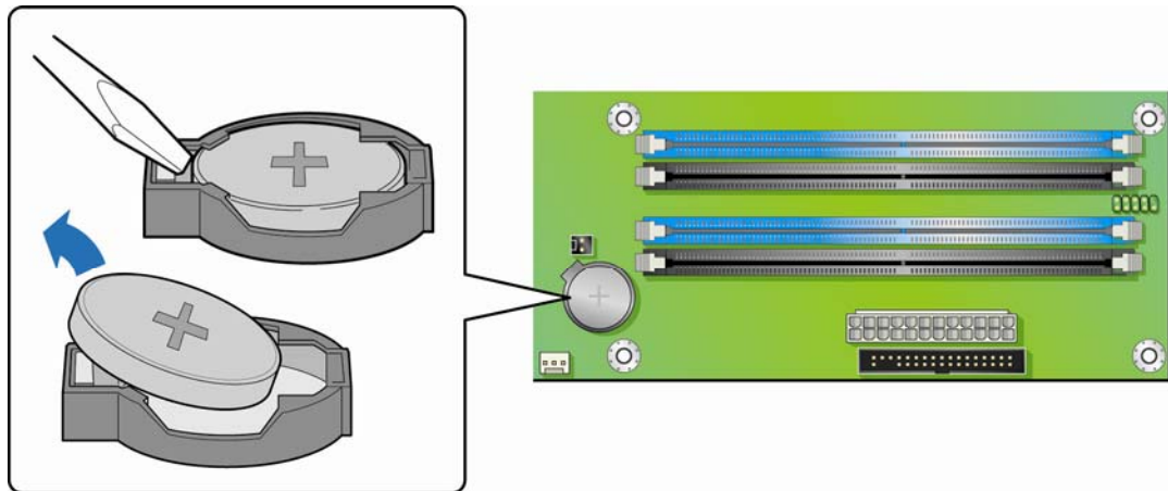
图 29. 拆卸电池
