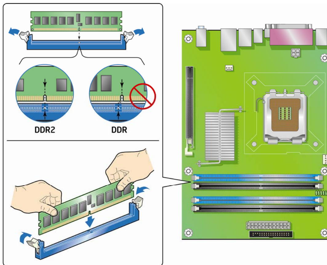
图 17. 安装 DIMM
