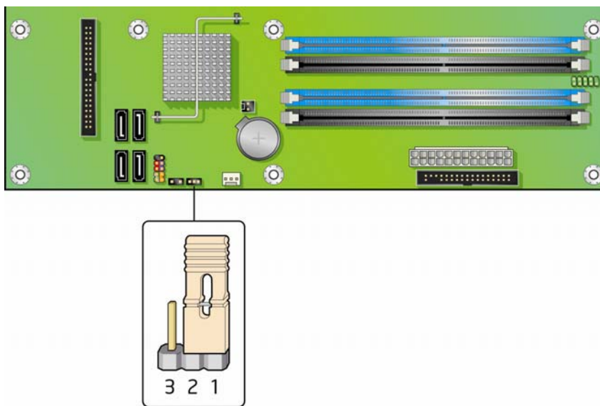
图 27. BIOS 配置跳线块位置
