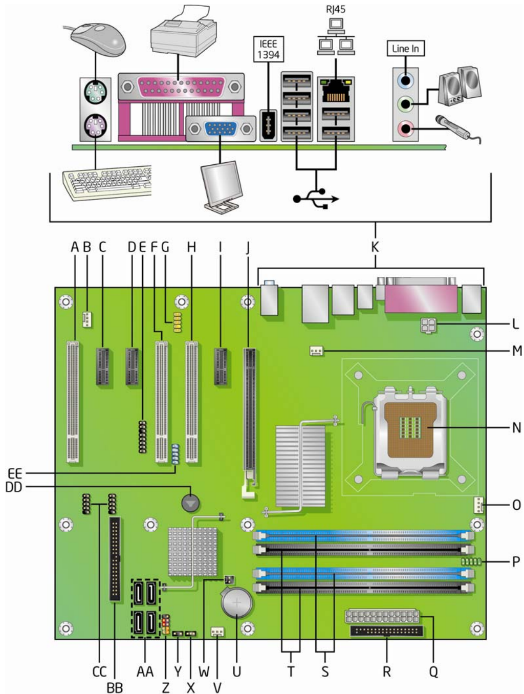
图 1. 台式机主板 DG965RY 组件
