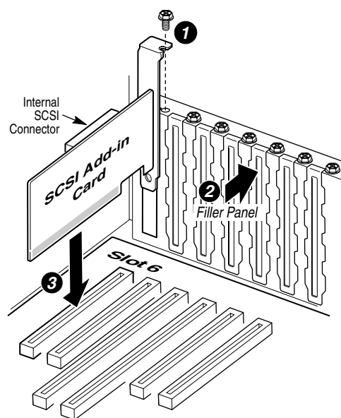
图 19. 安装附加卡
