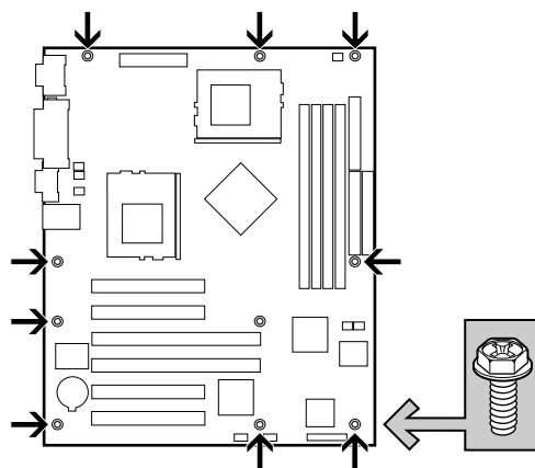
图 18. 固定服务器主板
