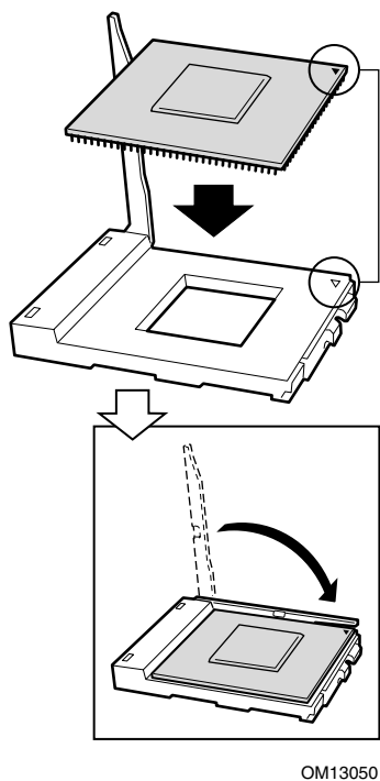
图 9. 插入处理器
