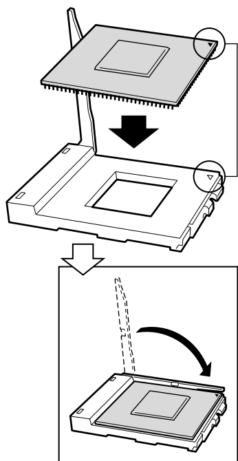
图 26. 插入处理器
