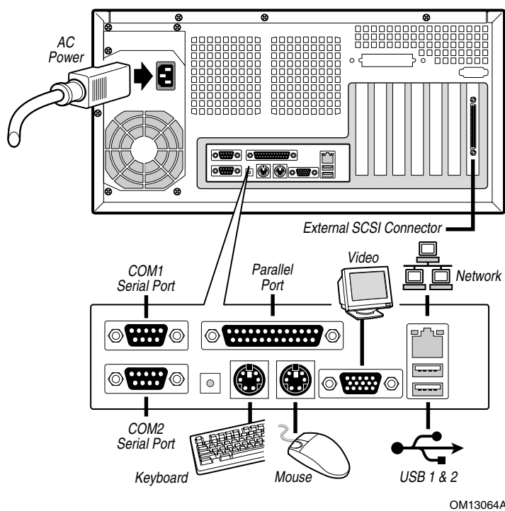
图 23. 背面板连接
