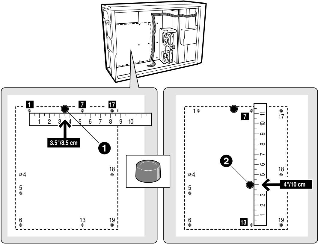
图 15. 安装防震橡胶垫
