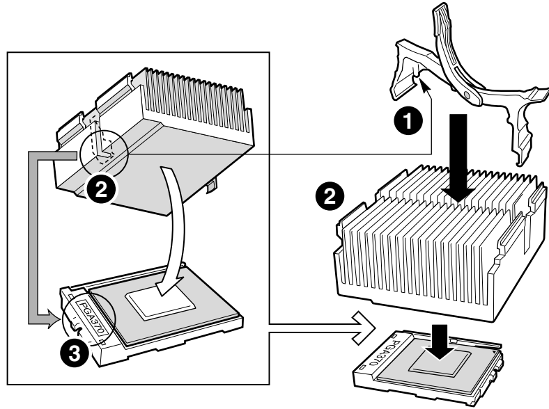
图 27. 连接散热器固定夹
