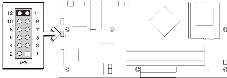
图 31. 配置跳线的位置
