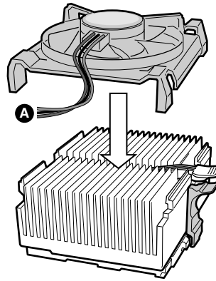
图 29. 连接散热器风扇
