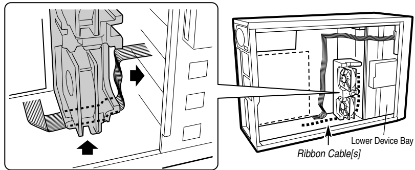
图 21. 布线 IDE 或 SCSI 电缆
