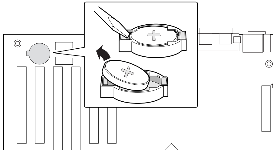
图 30. 更换备用电池
