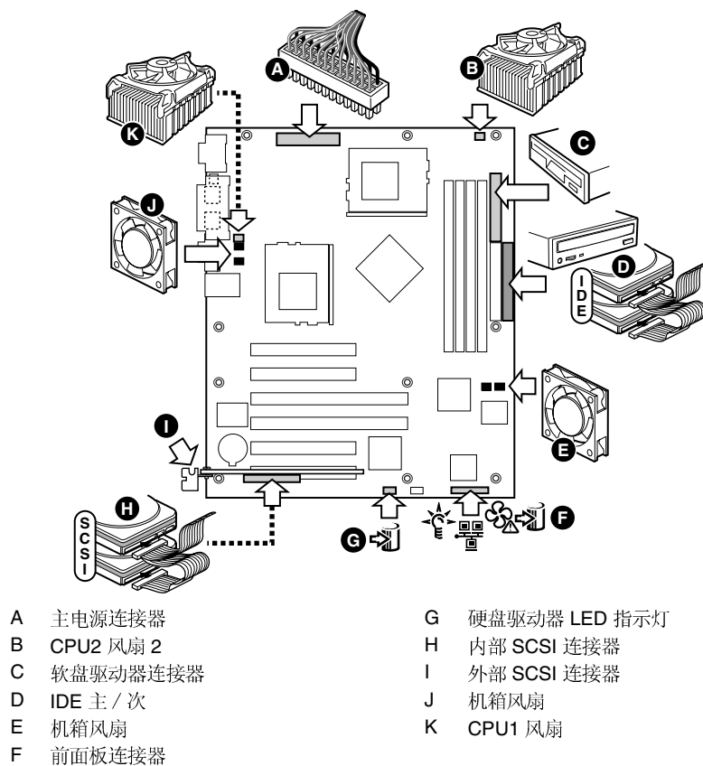
图 20. 连接至服务器主板
