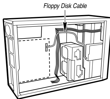
图 22. 布线软盘驱动器电缆
