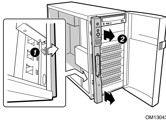
图 3. 拆卸前护盖
