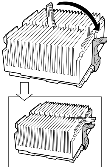
图 28. 锁定散热器固定夹
