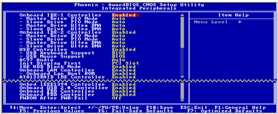
圖 3-7. 整合週邊設定選單畫面
