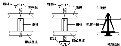
圖 2-2. 固定主機板至機殼的幾種方法
