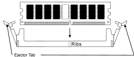
圖 2-4. 安裝記憶體模組
