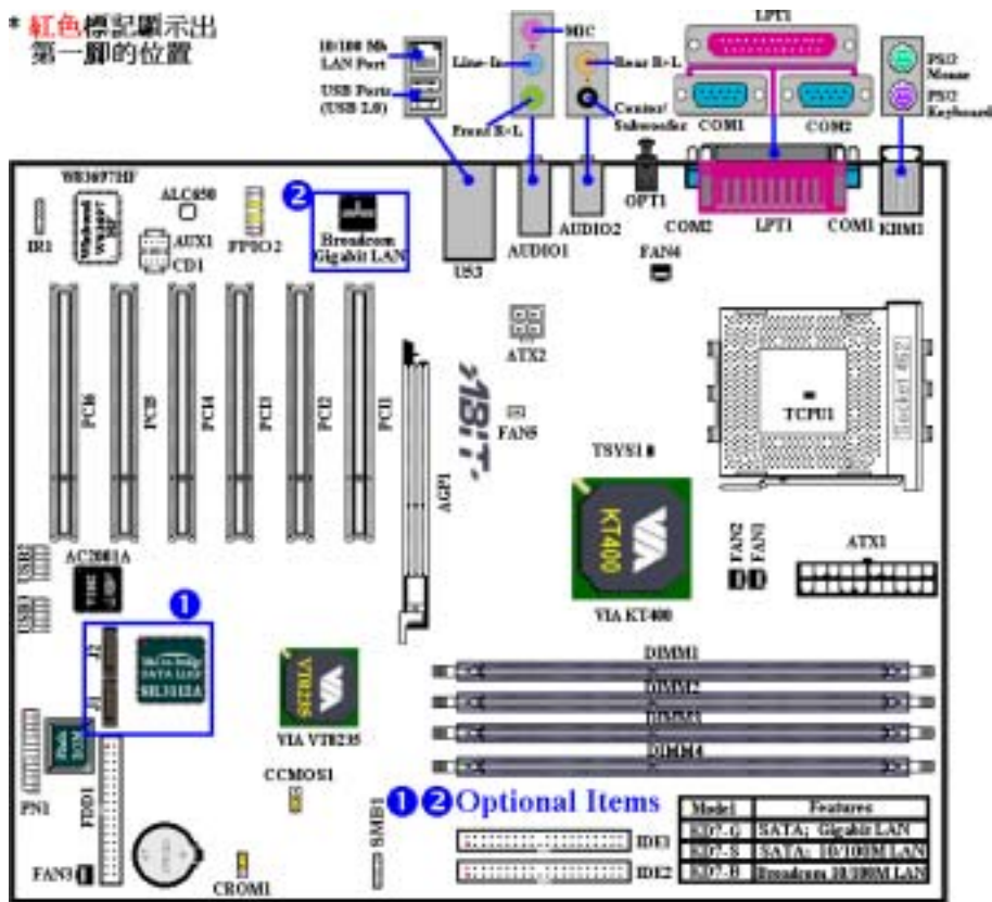
圖 1-1. KD7-B/KD7-S/KD7-G 主機板重要元件位置圖
