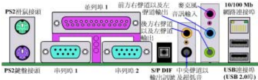
圖 2-9. KD7-B/KD7-S/KD7-G 背面面板的連接埠
