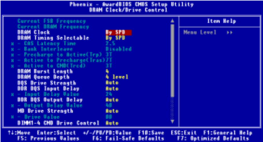
圖 3-5B. DRAM 時脈/驅動方式 控制選單的上半部畫面
