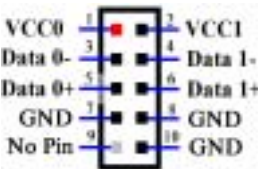
USB2/USB3
