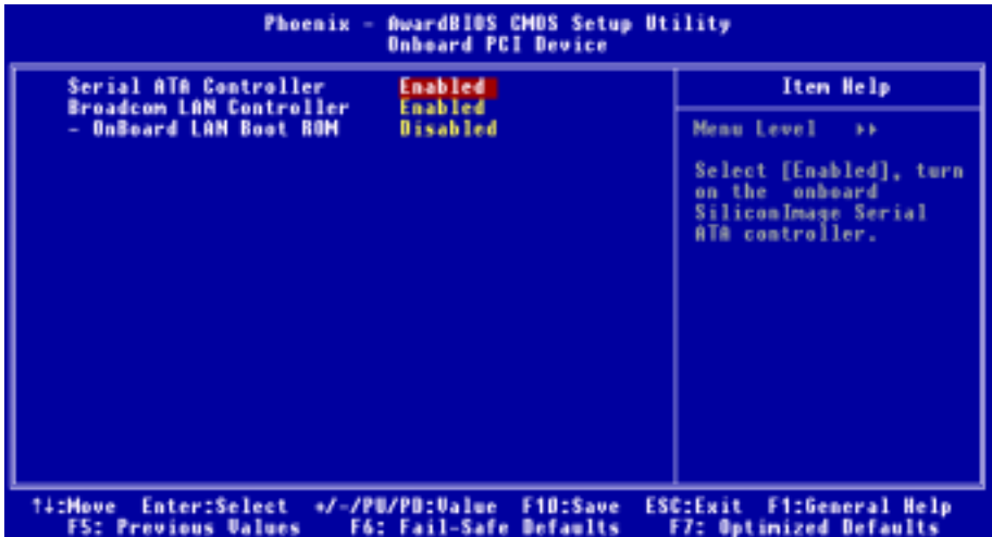
圖 3-6E. 主機板內建的 PCI 裝置設定畫面
