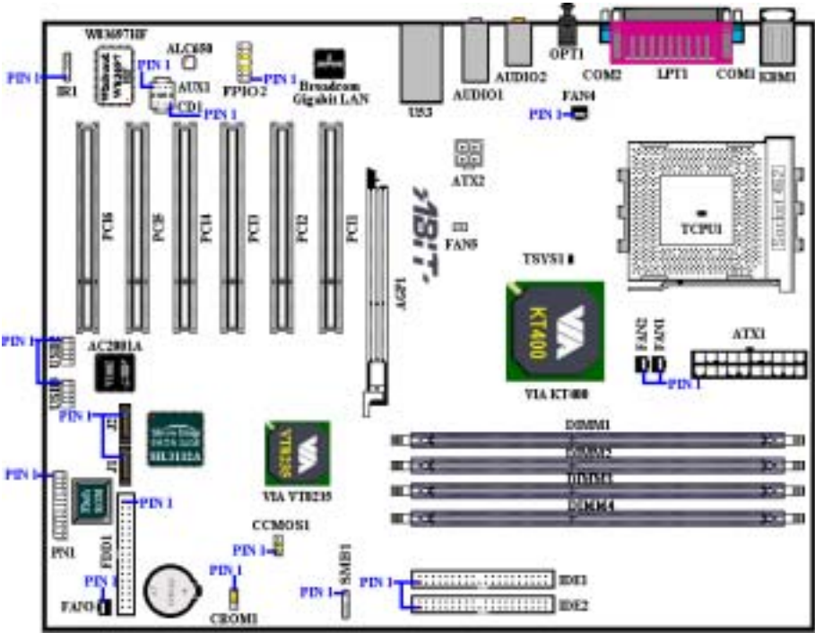
圖 2-7. KD7-G 主機板的所有連接埠和接頭
