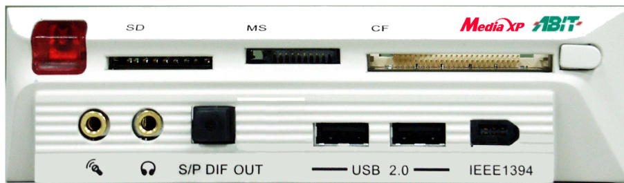
圖 1-1. ABIT Media XP/Media XP Pro 裝置的前面板照片
