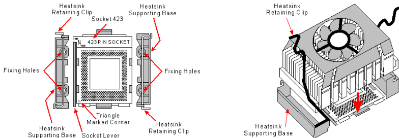
Abbildung 2-3. Installation der P4 CPU und ihres Kühlblechs in die Halterung.
