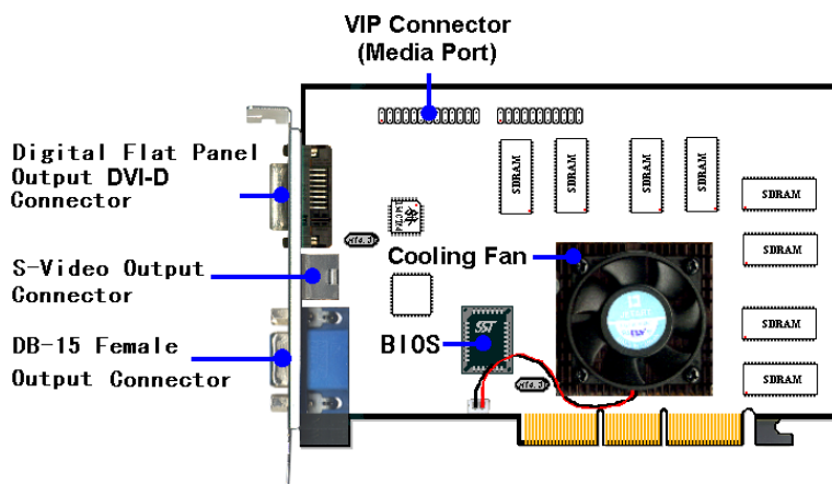
圖 2-2. SILURO™ GF256 重要零組件配置圖
