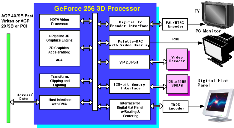
圖 2-4. SILURO™ GF256 顯示卡的系統方塊圖
