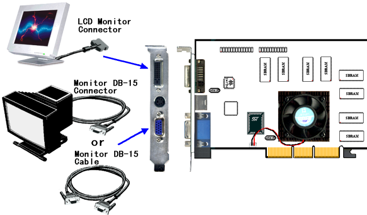
圖 2-6. SILURO™ GF256 至數位平面顯示器的連接
