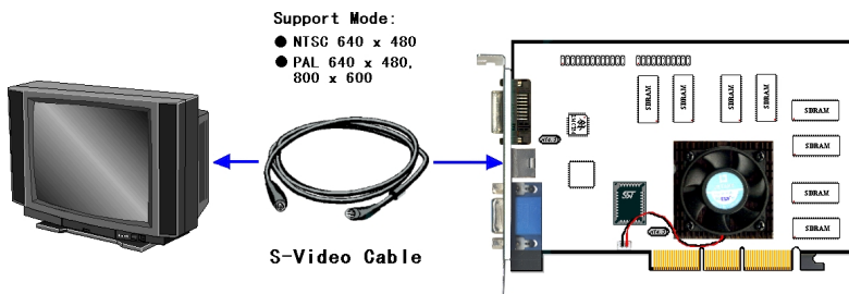
圖 2-5. SILURO™ GF256 至 TV 的連接方式
