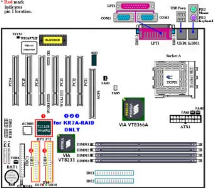
Abb. 1-1. Komponentenplan des KR7A/KR7A-RAID Motherboard
