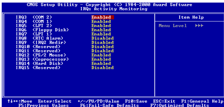
圖 3-7D. IRQ活動監視的設定選單
