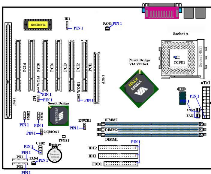
圖 2-7A. KT7 所有的連接埠及接頭
