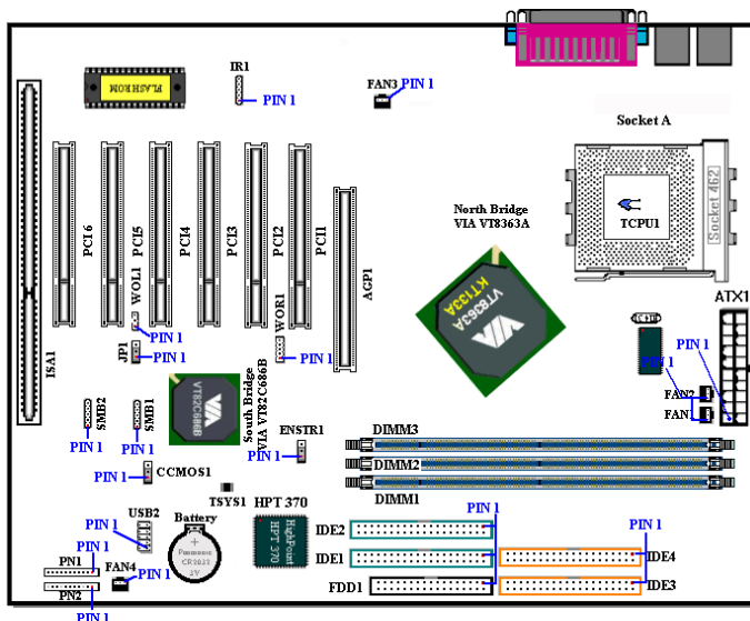
圖 2-7D. KT7A-RAID 所有的連接埠及接頭
