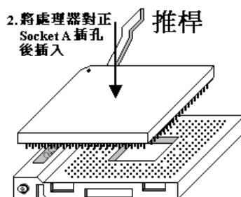
圖2-4. 將處理器安裝至Socket A之中
