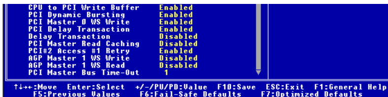
圖 3-5B. 晶片組進階功能參數設定選單下半部畫面
