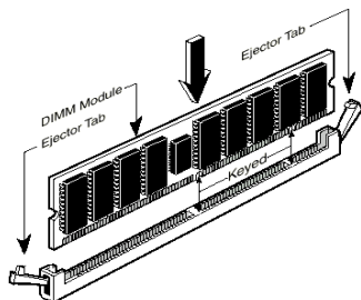
圖 2-6. 記憶體模組之安裝
