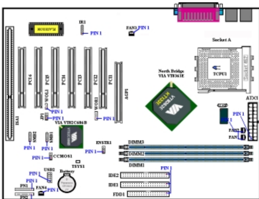
Figure 2-7. Tous les connecteurs et Switches de la KT7E
