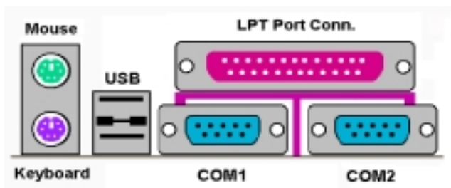
Figure 2-11. Connecteurs du panneau arrière de la KT7E
