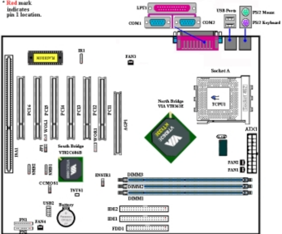
Figure 1-1. Emplacement des composants sur la KT7E
