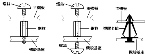
圖 2-2. 固定主機板至機殼的幾種方法
