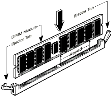
圖 2-6. 記憶體模組的安裝
