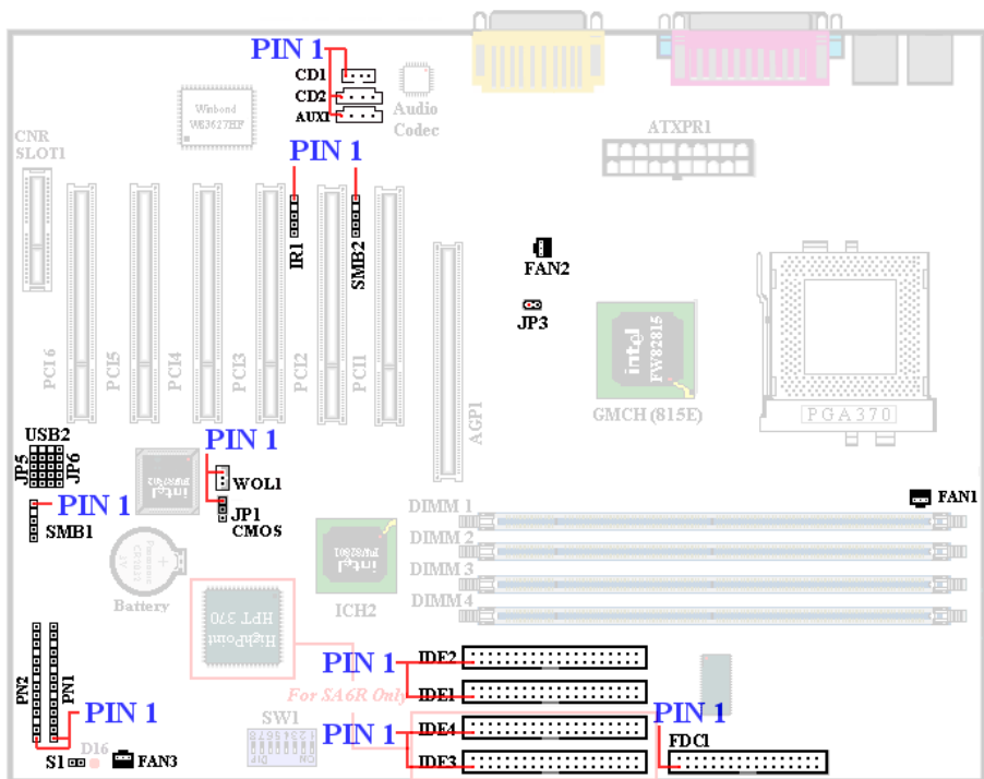
圖 2-7. SA6/SA6R 所有的連接埠及接頭
