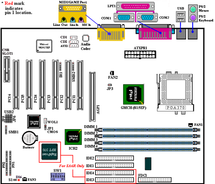
圖 1-1. SA6/SA6R 主機板重要元件位置圖
