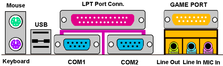
圖 2-11. SA6/SA6R 背板之連接器
