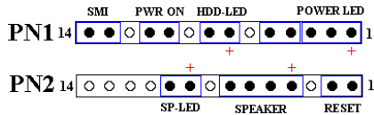
圖 2-9. PN1 與 PN2 針腳的定義
