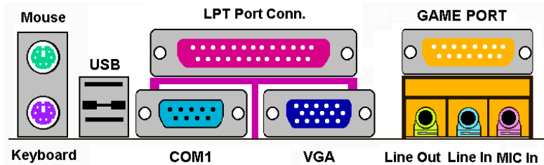
図 2-11. SE6 のバックパネルのコネクタ
