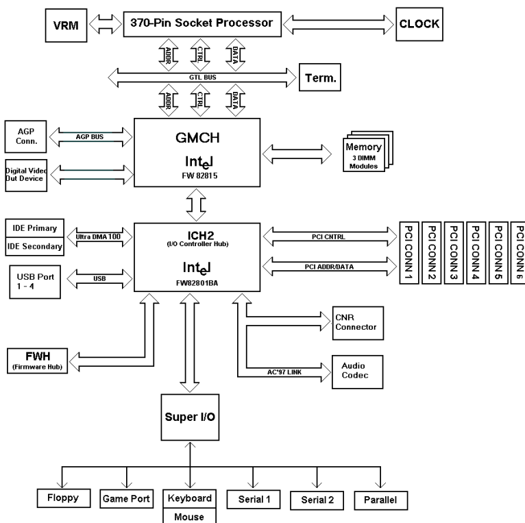
図 1-4. SE6 のシステムブロック図
