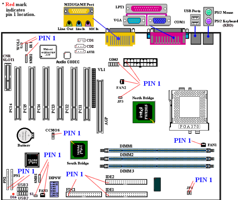
図 2-5. SE6 のコネクタとヘッダ
