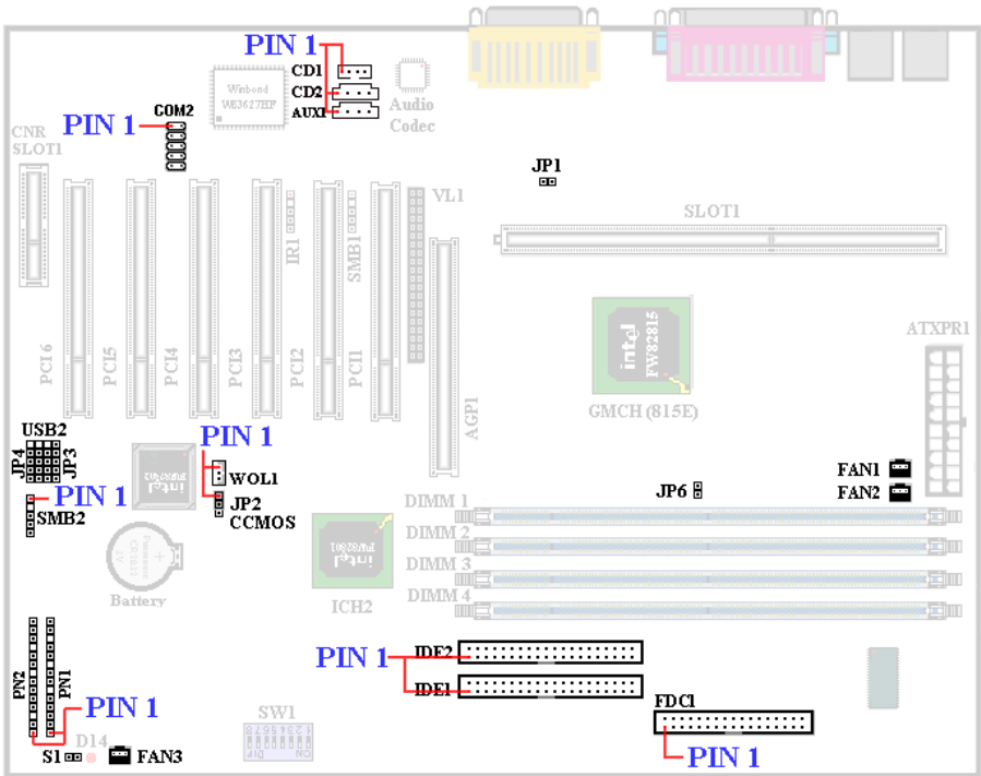
圖 2-5. SH6 所有的連接埠及接頭
