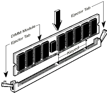
圖 2-4. 記憶體模組之安裝
