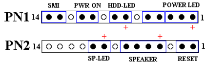
圖 2-9. PN1 與 PN2 針腳的定義
