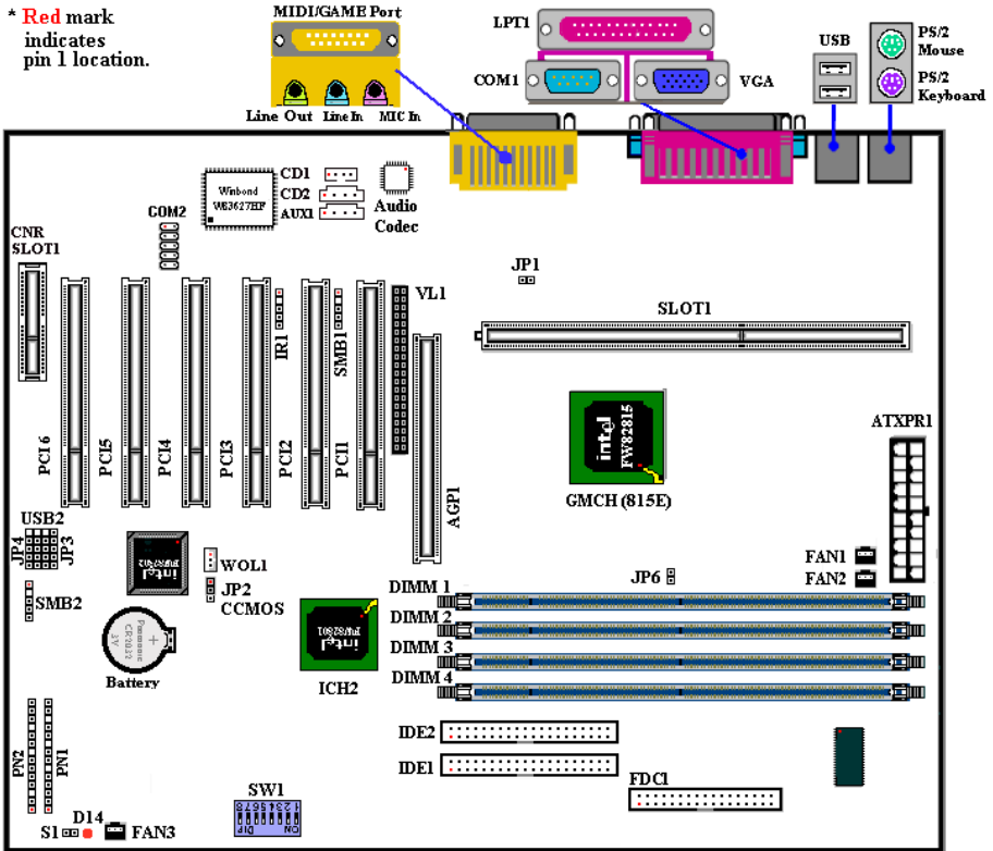
圖 1-1. SH6 主機板重要元件位置圖
