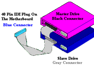
圖 2-8. 如何連接 Ultra ATA/66 的排線到主機板上
