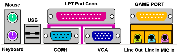
圖 2-9. 背板之連接器
