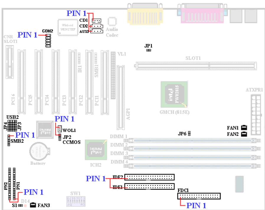
図 2-5. SH6 のコネクタとヘッダ
