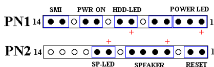
図 2-7. PN1 と PN2 の設定
