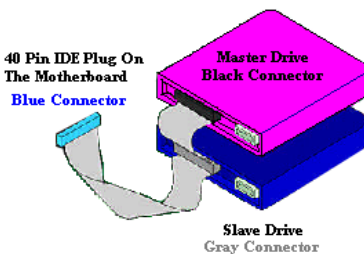
図 2-8. Ultra ATA/66 ケーブルの接続方法
