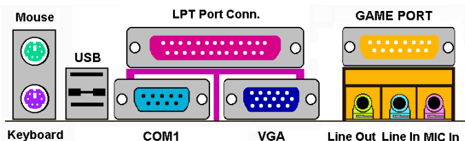
図 2-9. SH6 のバックパネルのコネクタ
