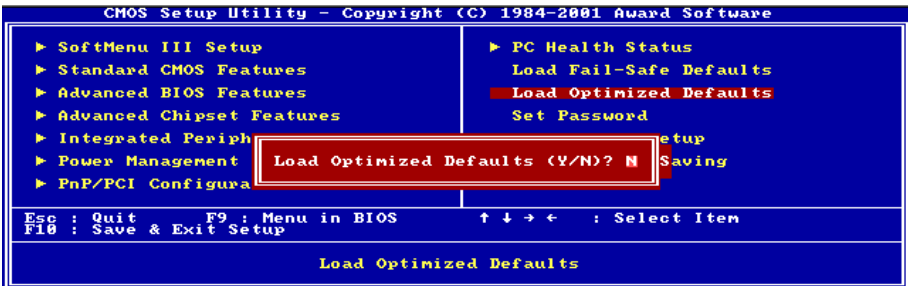
図 3-12. Load Optimized Defaults スクリーン
