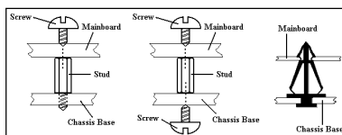
図 2-2. マザーボードを固定する方法
