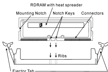
図 2-6. メモリモジュールの取付け
