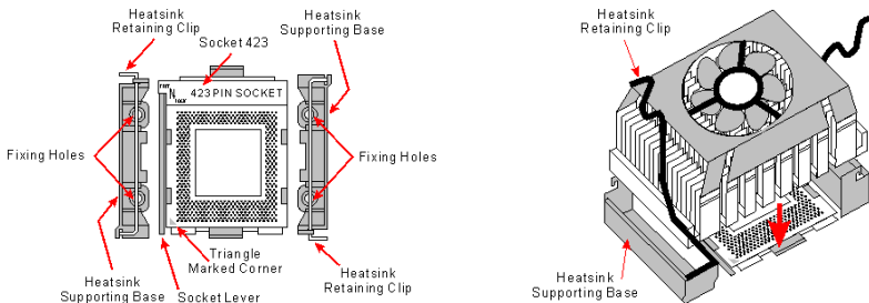
図 2-3. P4 CPU およびそのヒートシンクをサポート台に取り付ける。
