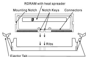
Abbildung 2-6. Speichermodul-Installation
