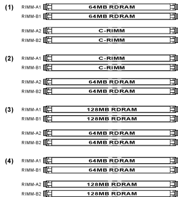
Abbildung 2-5. Beispiel für Speichermodul-Konfigurationen
