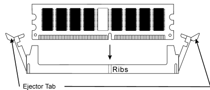
Figure 2-4. Installation du module de mémoire
