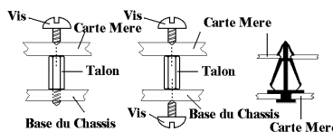
Figure 2-2. La manière de fixer la Carte Mère
