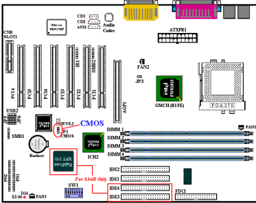
Figure 2-8. Paramétrage cavalier du JPI(CMOS)
