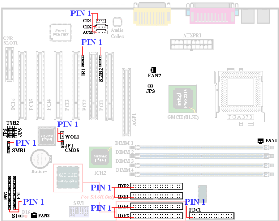
Figure 2-7. Dispositions de tous les connecteurs et broches sur la SA6/SA6R
