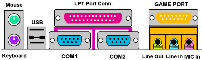
Figure 2-11. Disposition des connecteurs arrière de la SA6/SA6R
