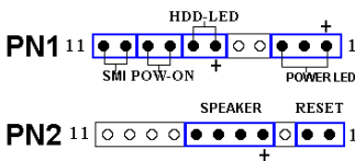
Figure 2-9. définitions des pins du PN1 et PN2
