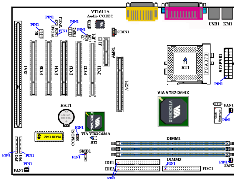
Figure 2-7. Tous les connecteurs de la VH6
