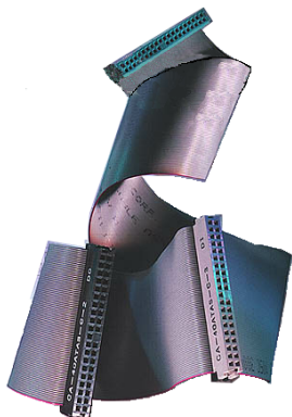
Figure 2-11. Photo d'une nappe Ultra ATA/66
