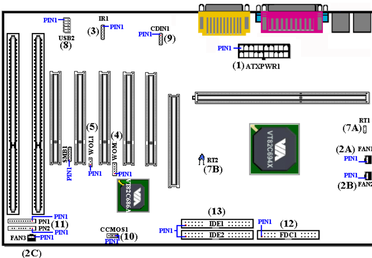
Figure 2-5. Tous les connecteurs de la VT6X4
