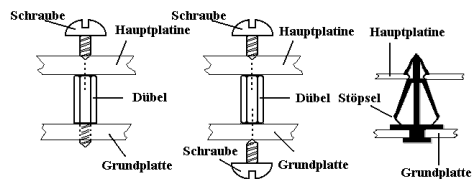
Abbildung 2-2. Befestigungsarten für die Hauptplatte
