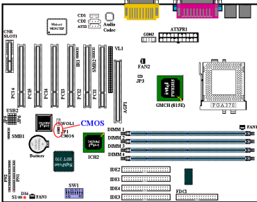
Abb. 2-8. JP1(CMOS)-Steckbrückeneinstellung
