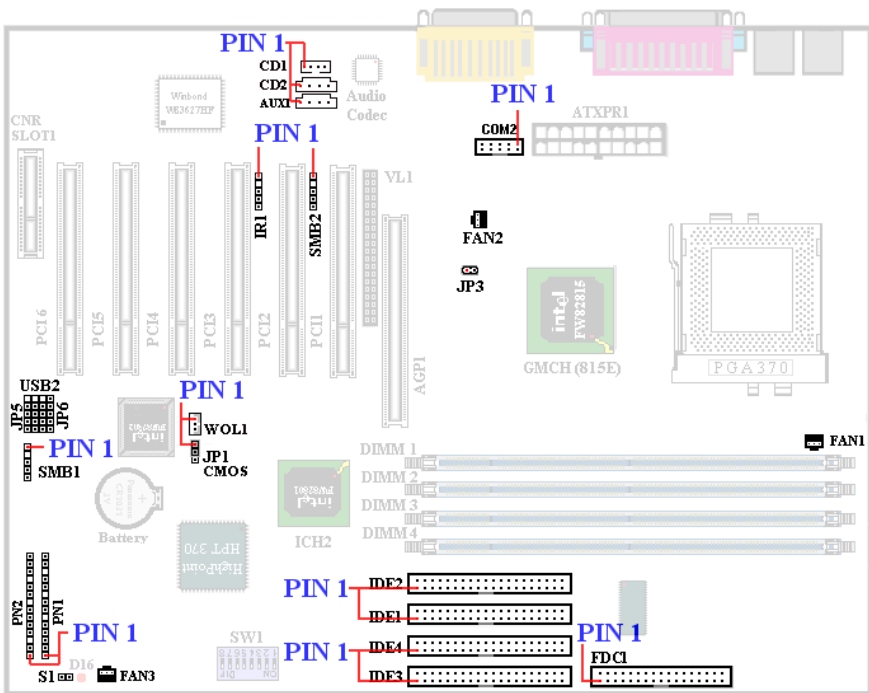
Abb. 2-7. Die Anschlüsse und Headers des SA6R
