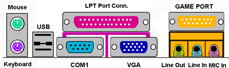
Abb. 2-11. Anschlüsse auf der Rückseite des SA6R
