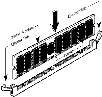
Abb. 2-6. Installation der Speichermodule
