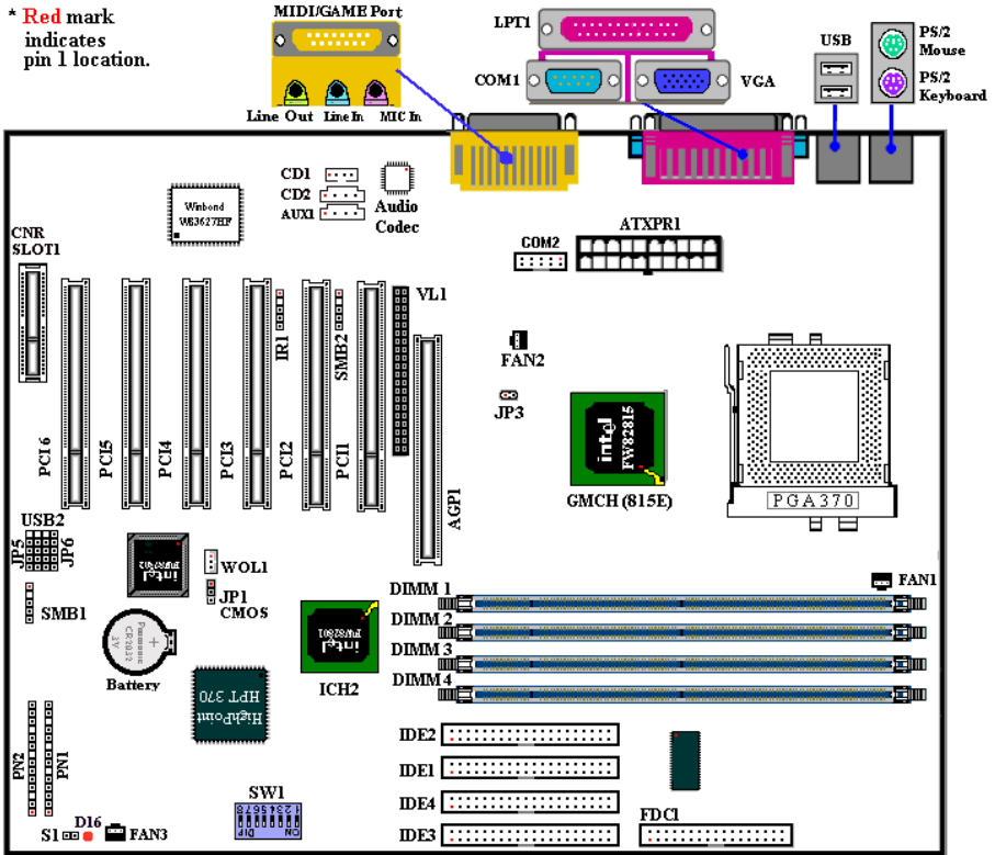
Abb. 1-1. SA6R Anordnung der Komponenten
