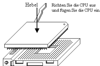
Abb.2.4 Installation der CPU in den Socket
