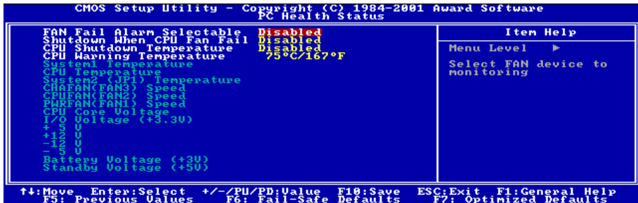
図 3-10. PC Health Status スクリーン
