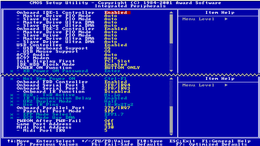
図 3-6. Integrated Peripherals Menu スクリーン
