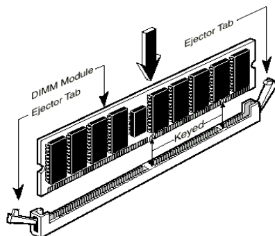
図 2-4. メモリモジュールの取付け
