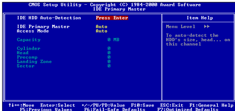
図 3-3B. IDE Primary Master Setup
