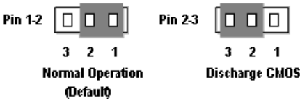
図 2-6 CCMOS ジャンパの設定
