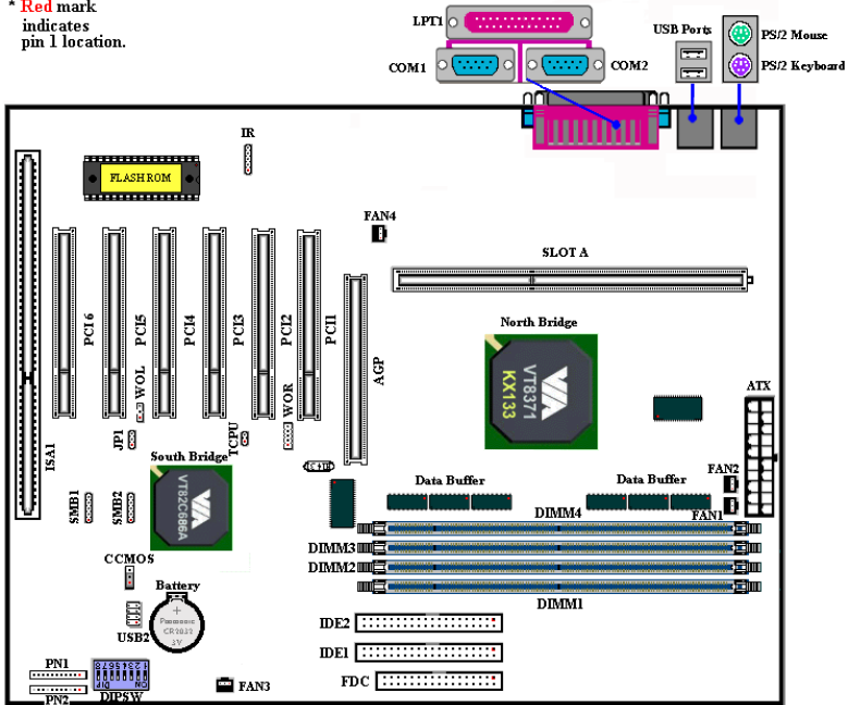
図 1-1. KA7 のコンポーネントの位置
