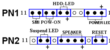
図 2-7 PN1 と PN2 の設定
