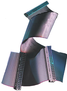
図 2-9 Ultra ATA/66 コンダクタケーブル
