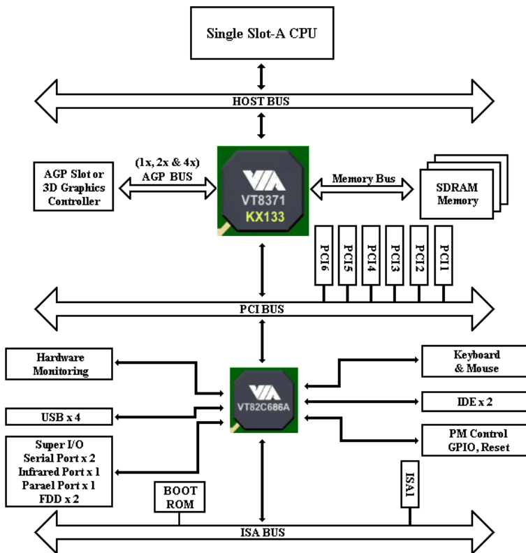
図 1-3. KA7 のダイアグラム
