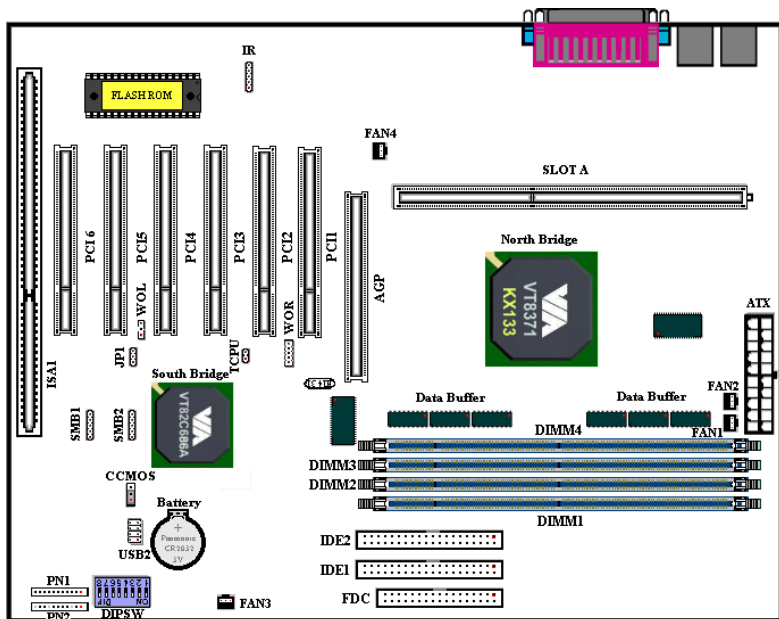
図 2-5 KA7 のコネクタとヘッダ
