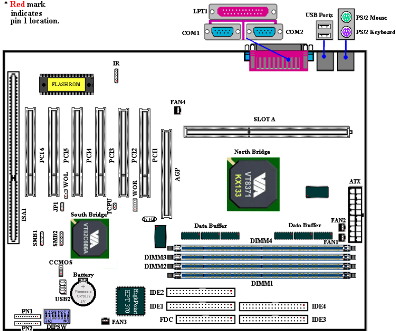
図 1-2. KA7-100 のコンポーネントの位置
