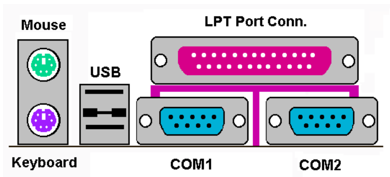
図 2-11 KA7/KA7-100 のバックパネルのコネクタ
