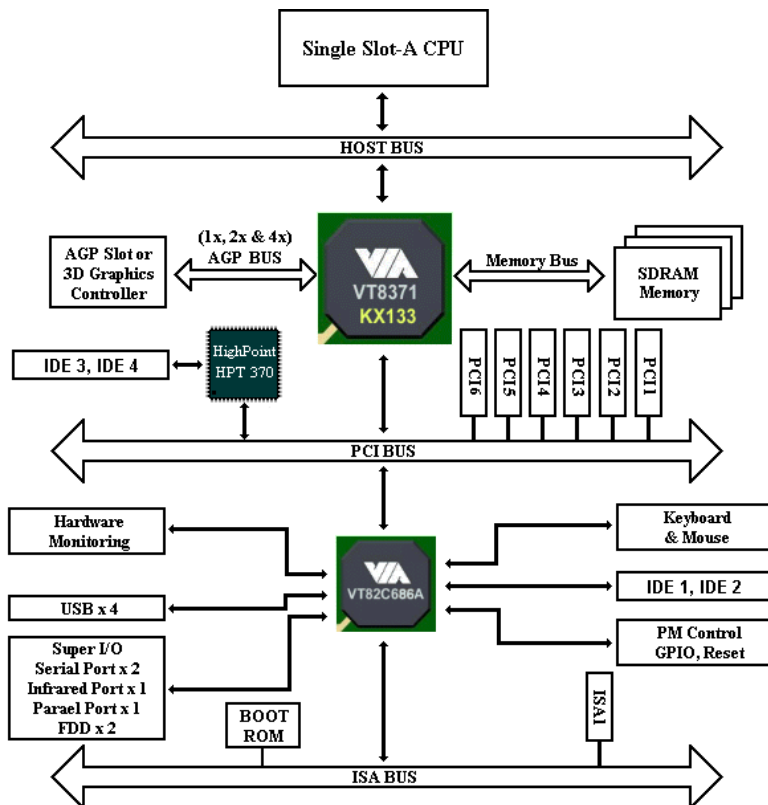
図 1-4. KA7-100 のダイアグラム
