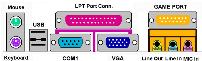
図 2-11. SA6R のバックパネルのコネクタ
