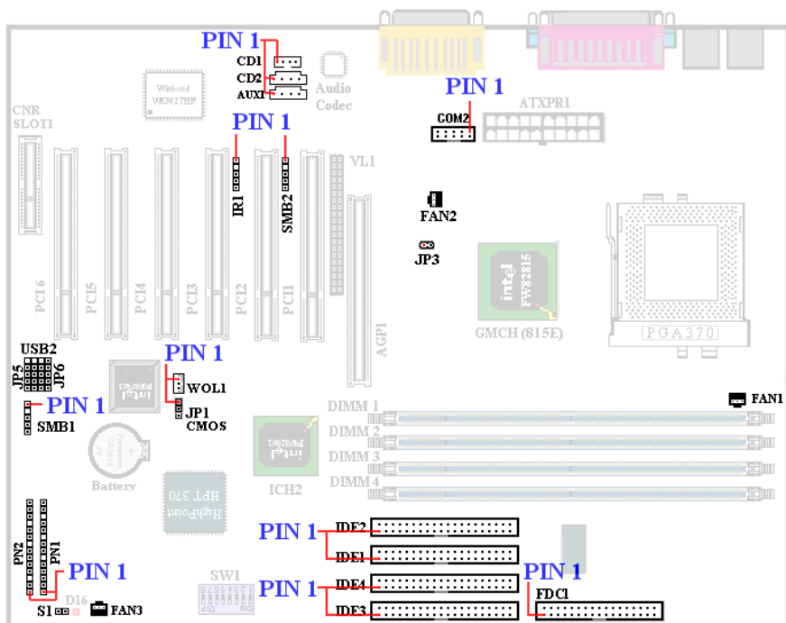
図 2-7. SA6R のコネクタとヘッダ
